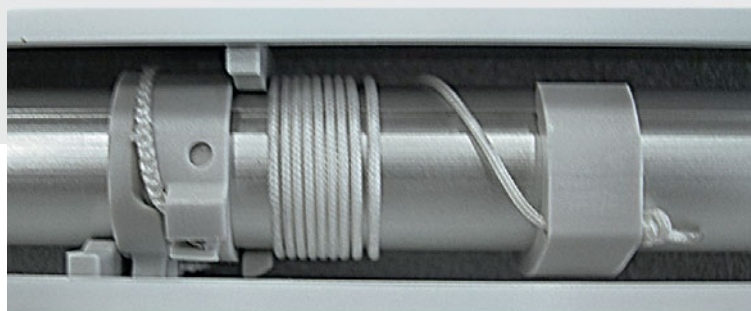
Particolari della meccanica
